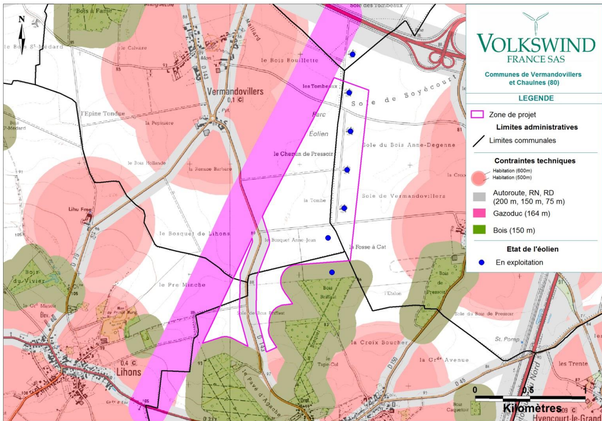
Carte 4 : Contraintes techniques du projet éolien
